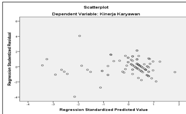
Gambar 3 Uji Heteroskedastisitas
