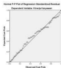
Gambar 1. Grafik Normalitas P-P Plot
